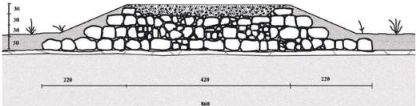
Estructura del terraplén de la vía romana en las Mijaradas , Burgos. © Isaac Moreno Gallo.
